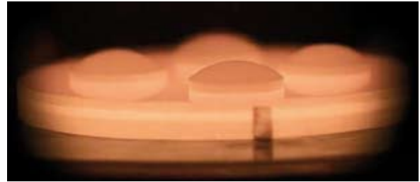
HEISSE SACHE: Die Technik der Gasphasenabscheidung (englisch Chemical Vapour Deposition, CVD) funktioniert nur unter enormen Temperaturen. An der rotglühenden Grundform, dem sogenannten Substrat, entstehen direkt aus Methangas künstliche Schichten kristallinen Diamants. Vier Kalotten wachsen hier gleichzeitig, deren Form schon erahnbar ist.
